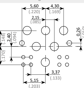
Module à picots soudés Module with angled PCB contacts
