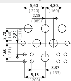
Module à picots droits Module with straight PCB contacts
