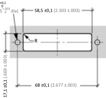
Montage par l'arrière (pour PCB) Rear mounting (for PCB)
